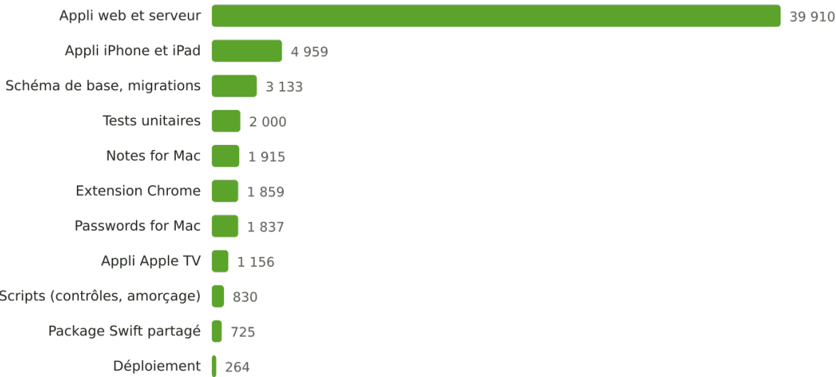
Lignes de code non vides par partie de Hearth (58 588 au total)
